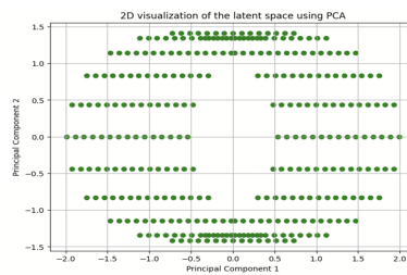
PCA
