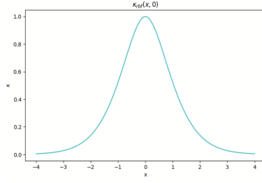
Matérn 5/2 kernel
