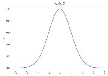
RBF kernel
